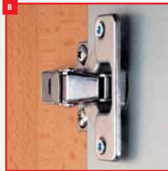
Рис. В: Обычный шуруп для древесностружечной плиты: безтормозное проворачивание шурупа на обшивке разрушает сопряженную резьбу в материале основания, обшивка отстает.
