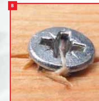
Рис. В: Обычный шуруп для древесностружечной плиты: расщепление при утапливании головки.
