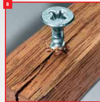
Рис. В: Обычный шуруп для древесностружечной плиты: расщепление древесины при заходе.
